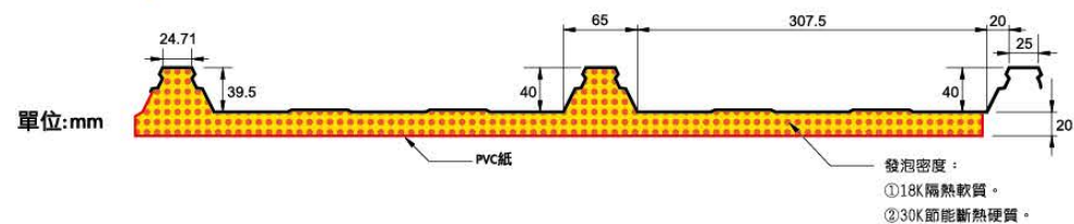
雙層斷面圖
