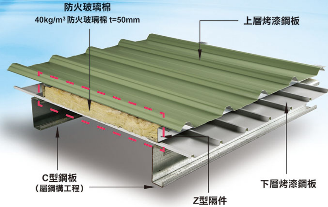
防火玻璃棉
