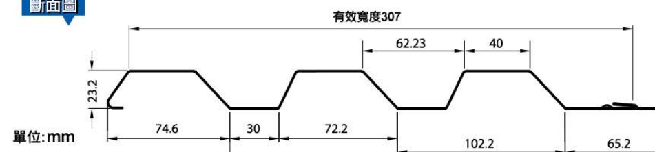
斷面圖
