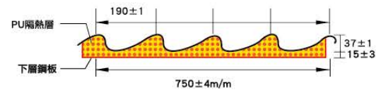
琉璃鋼瓦系列背面材質-白色烤漆鋼板
