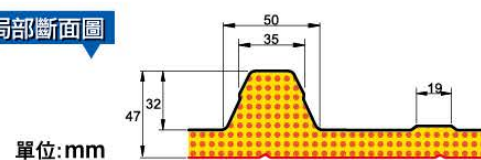
雙層斷面圖
