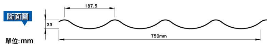
雙層斷面圖
