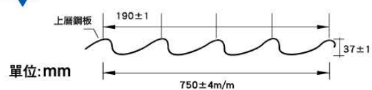
斷面圖
