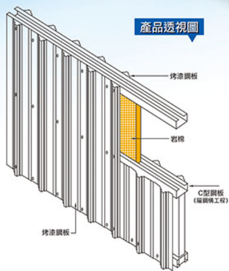
防火外牆組合圖
