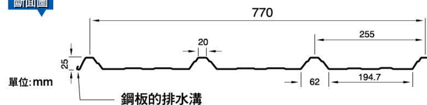
斷面圖
