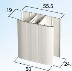
HY-02 (工字連接條組合)
