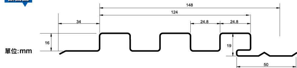
斷面圖
