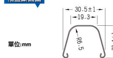
帽蓋斷面圖
