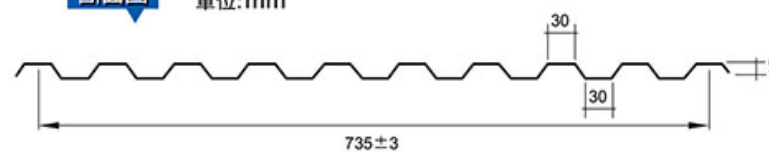
斷面圖
