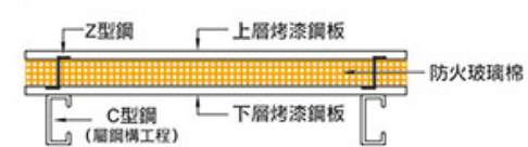
斷面圖
