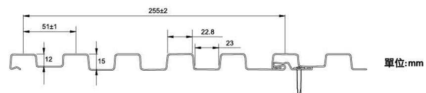
組合示意圖
