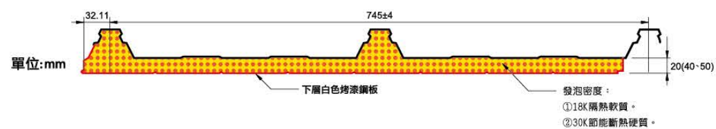
雙層斷面圖
