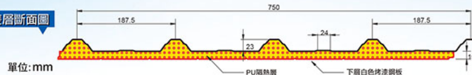
屋簷端蓋
