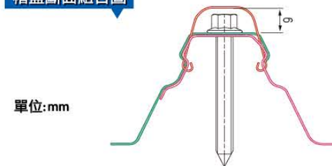
帽蓋斷面組合圖
