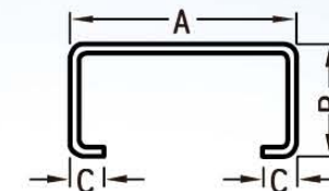
變形金剛 C型鋼 - 斷面圖
